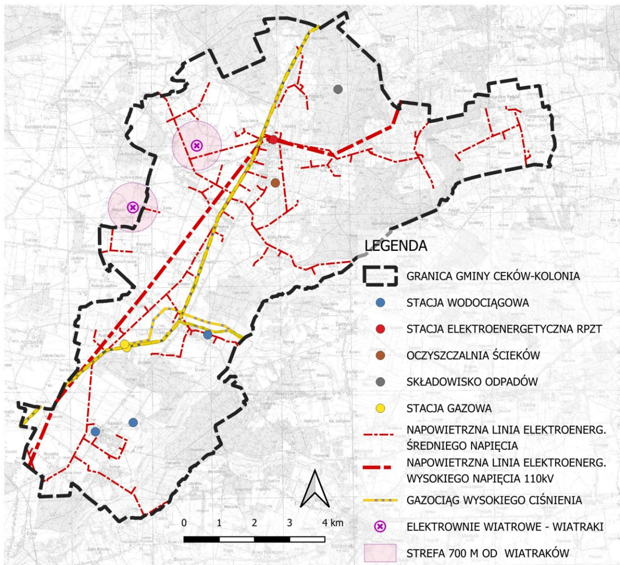
Rys. 11. Rozmieszczenie sieci infrastruktury technicznej
