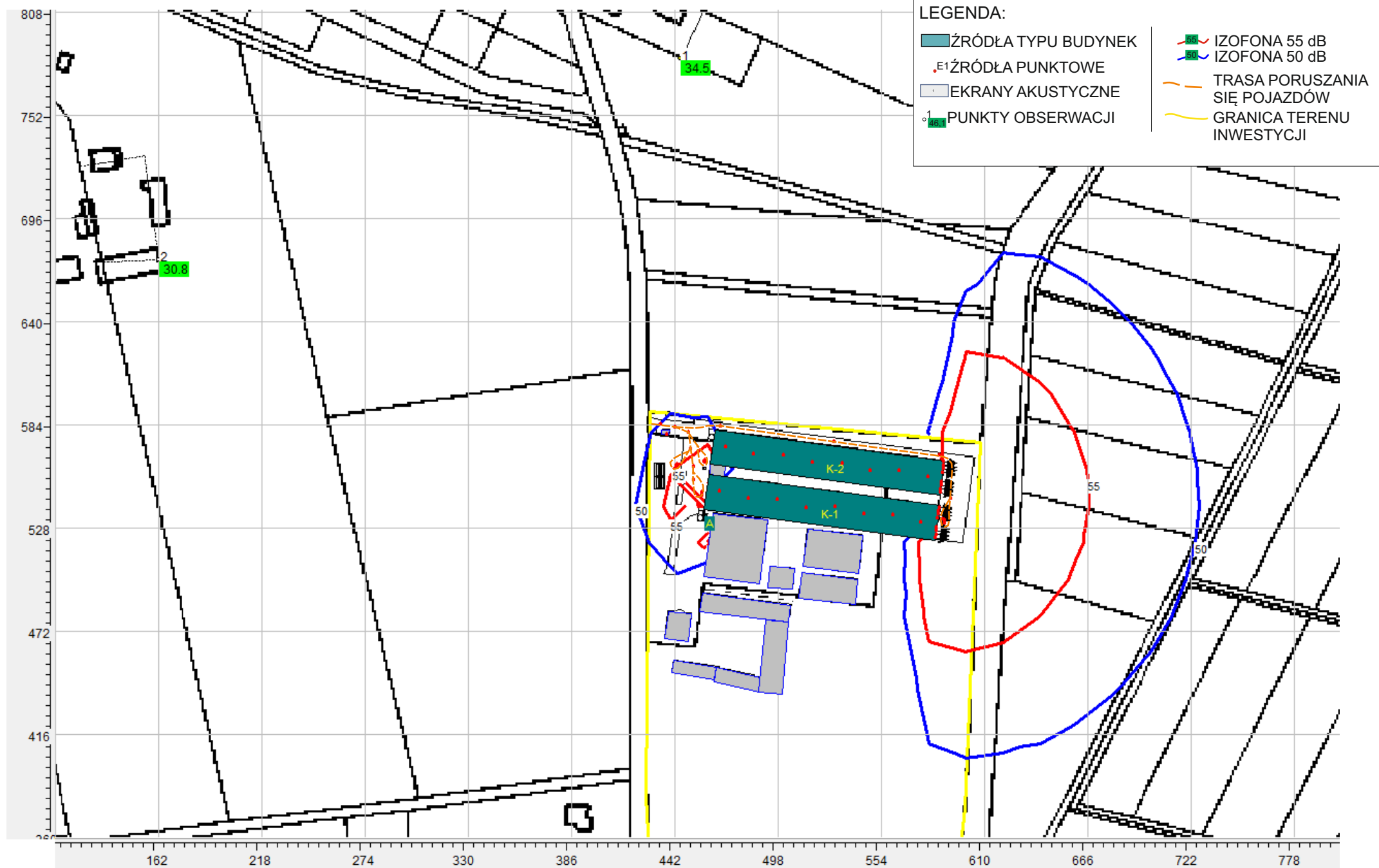
MAPA ROZKŁADU IZO FON - PORA DZIENNA
