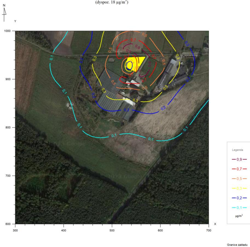
Izolinie stężeń średnich pyłu zawieszonego PM 2,5 µg/m 3
