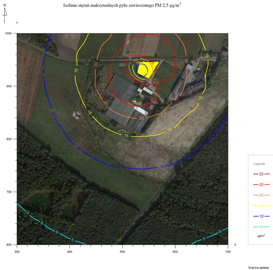
Izolinie stężeń maksymalnych pyłu zawieszonego PM 2,5 µg/m 3
